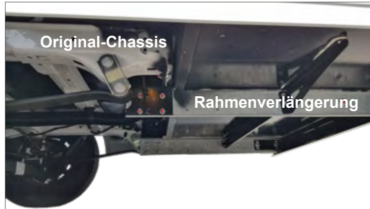
Verbindungsstelle vom Original- Chassis zur Rahmenverlängerung
